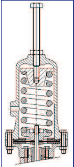
Actuator 100/120
